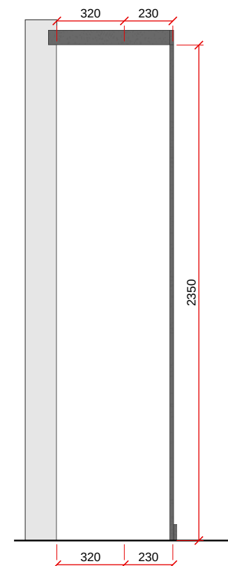
VISTA A - LATERAL - ESC. 1:25
