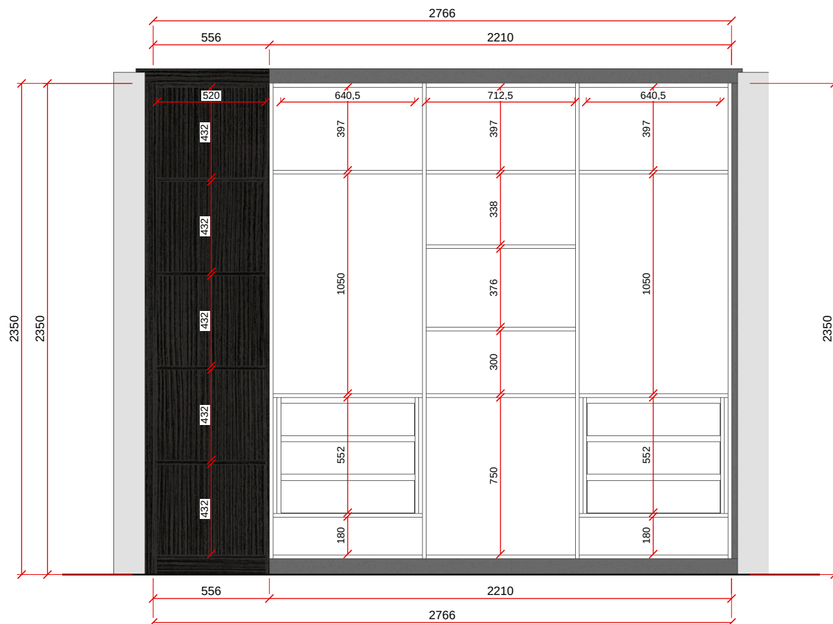
VISTA A - ESC. 1:25
